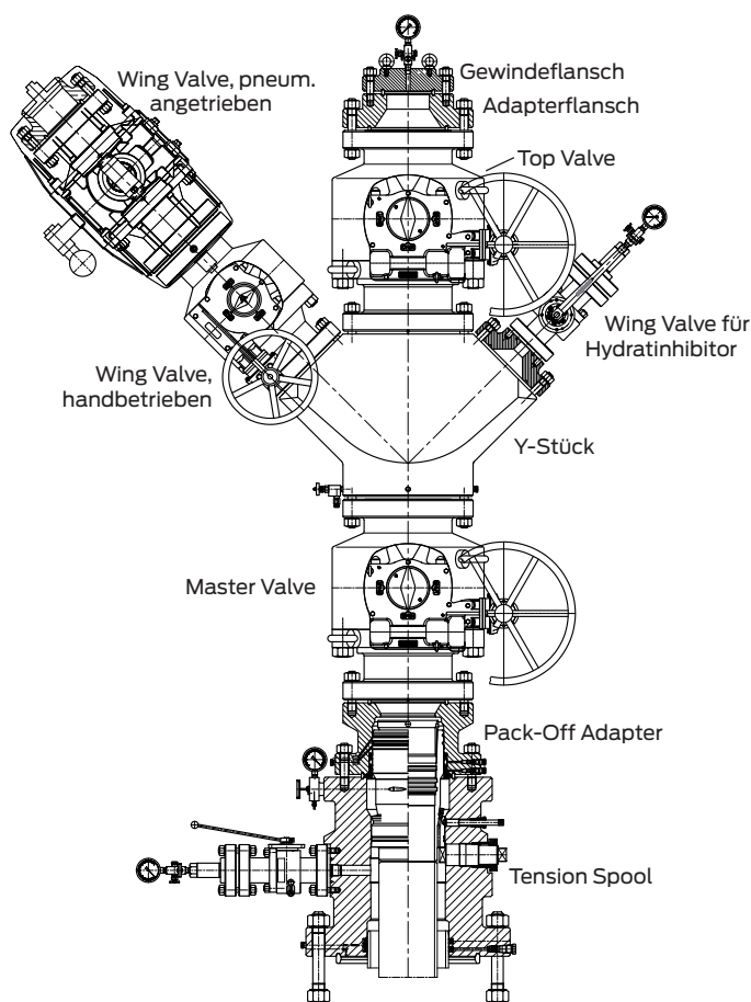
Hartmann Wellhead für den Gasspeicherbetrieb
